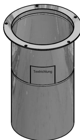
Abb. 52: Einschubadapter zur Montage auf bestehenden Rauchaasanlagen
