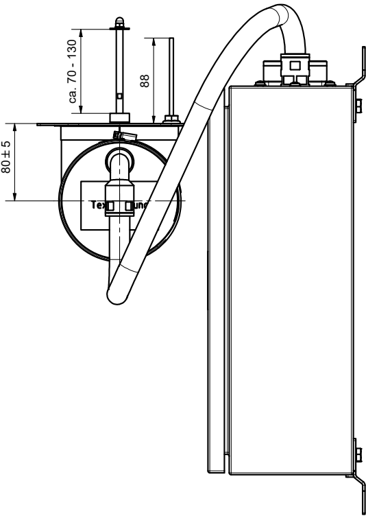
Abb. 43: Maße Ansicht 3 Partikelabscheider Airjekt 1 Outdoor (Draufsicht)
