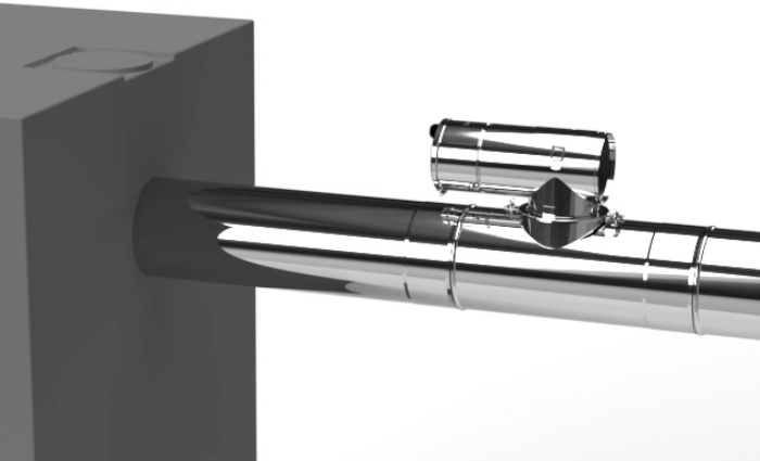
Abb. 19: Einbaurichtung horizontal
