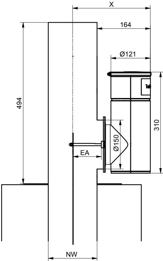
Einbau top
