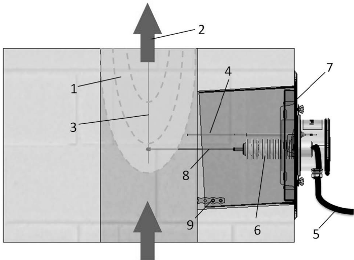
Abb. 30: Baugruppenübersicht Abscheidereinsatz (Airjekt 1 Ceramic mit RS-Türuns Schachtverlängerung)
