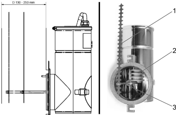
Abb. 21: Elektrode (1), Keramikisolator (2), Verschiebesicherung (3)
